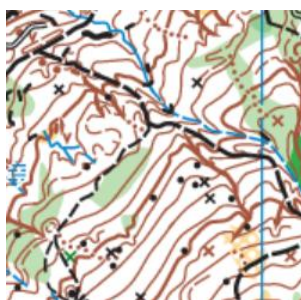
Bedero – Valcuvia
